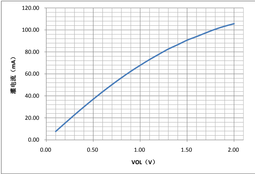
(5) 低电平驱动能力 ( V_{DD}=5V )
