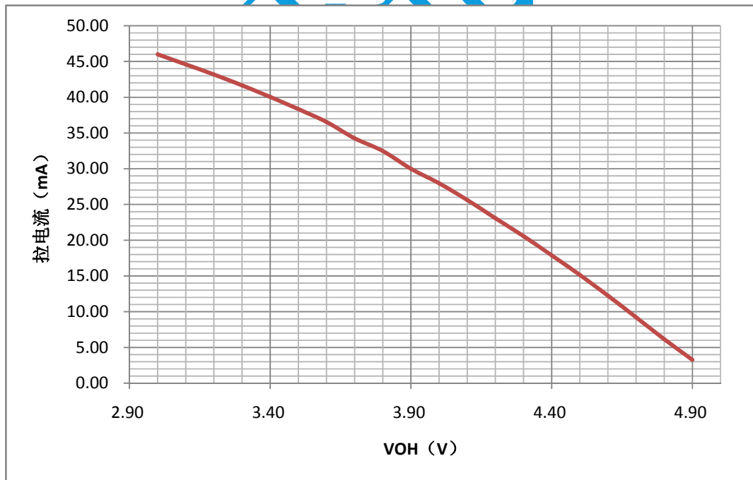
(4) 高电平驱动能力 (VDD=5V)
