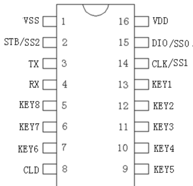
图 5-1 GRM807FNS_0B 管脚图
