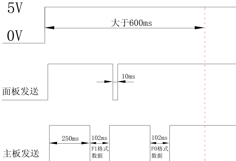
图 10-1 逻辑时序
